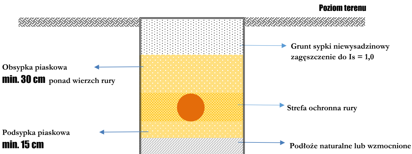
Rysunek 1: Układanie rur kanalizacyjnych w wykopie.
